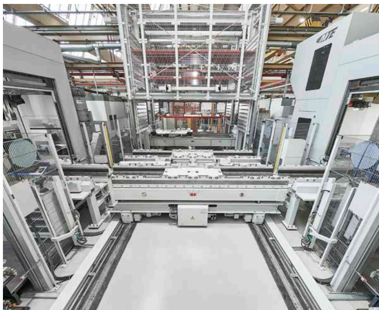
Doppelbeladedrehtisch zur Bestückung der CNC-Bearbeitungszentren
